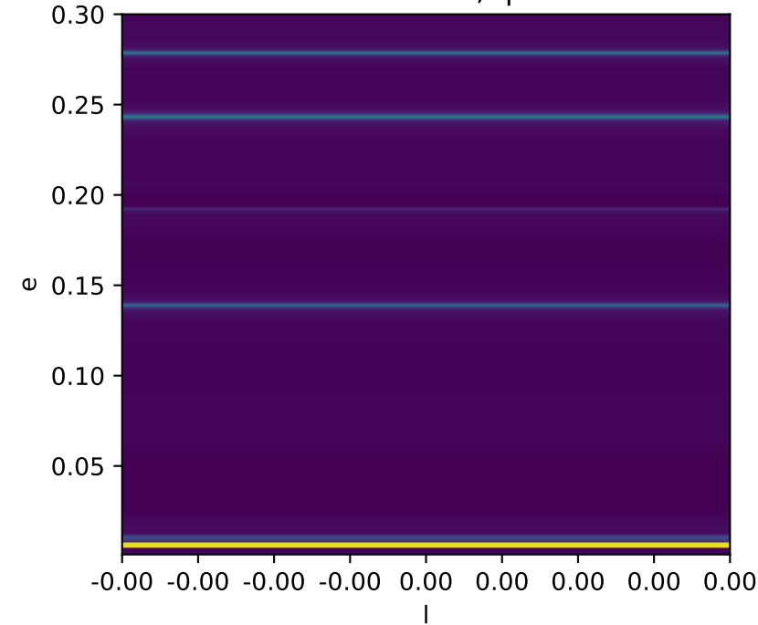
k=Iso \nu=2.5 , q=1
